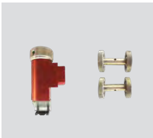
KIT B - FLM110 Pelado de cubierta de capa semiconductora
