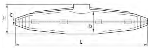
Dimensiones
