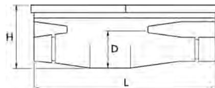
Dimensiones
